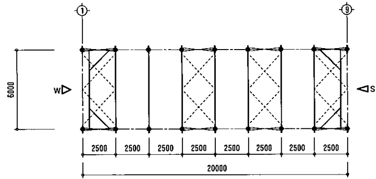
基礎伏図 S=1/200
