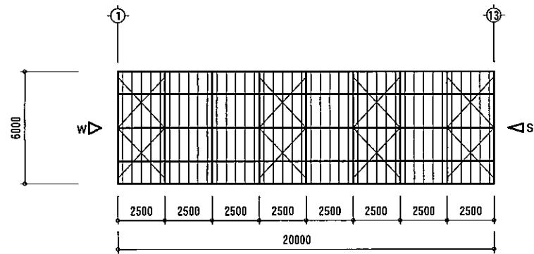
小屋伏図 S=1/200
