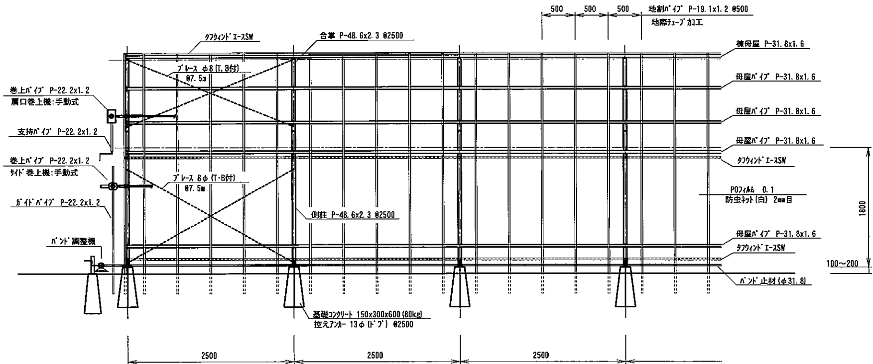
側通り立面図
