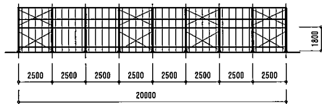
側立面図 S=1/200
