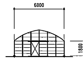
9通り 妻立面図 S=1/200
