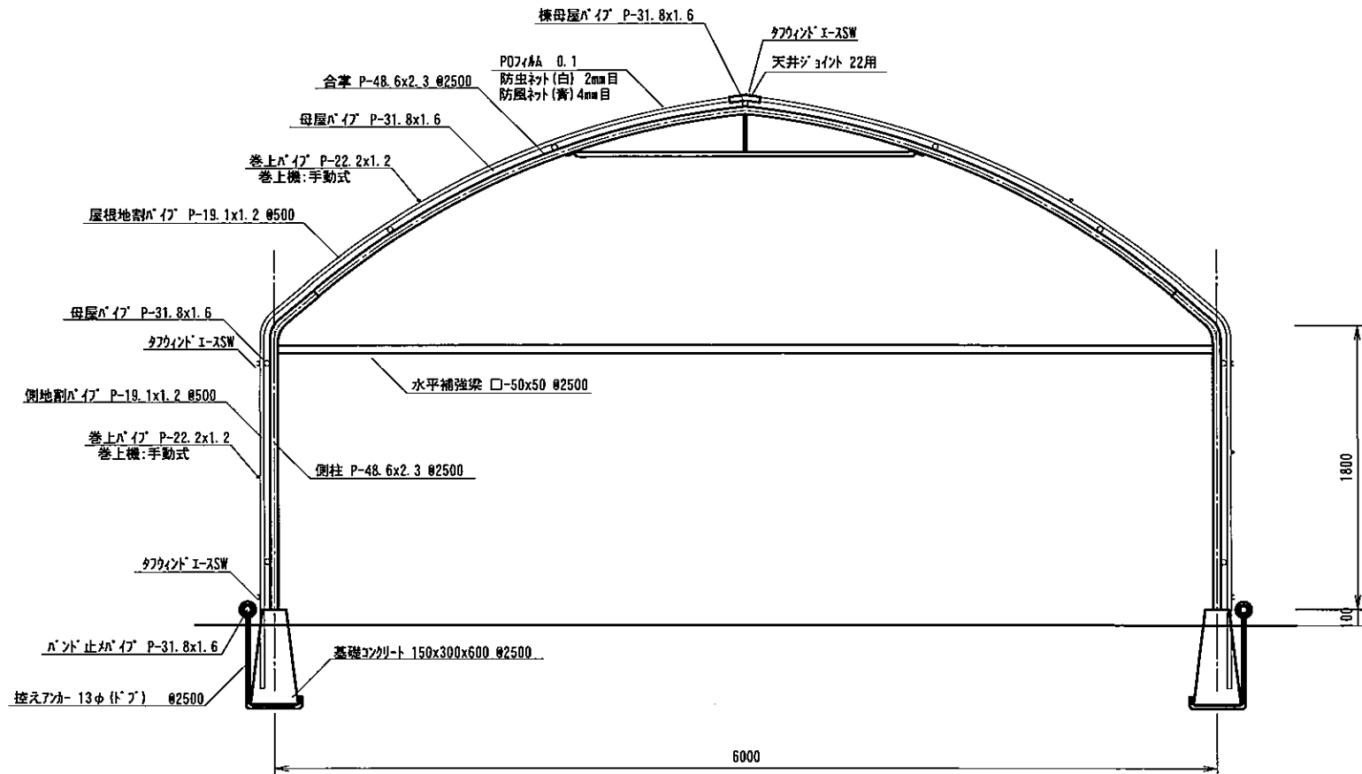
矩計図
