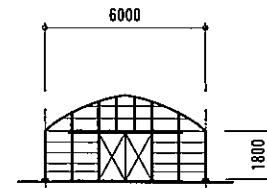
1通り 妻立面図 S=1/200
