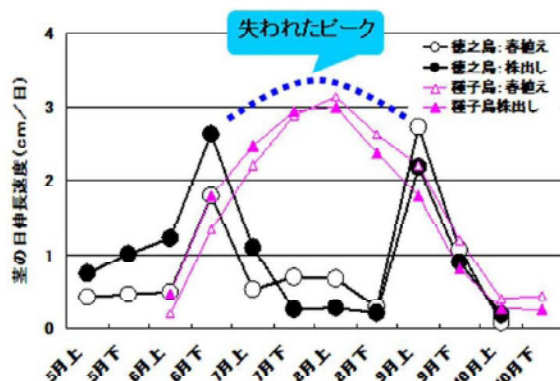
▼サトウキビの茎伸長速度の推移（2006 年。○春植え、●株出し）
