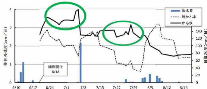
▼2016 年夏の降水量およびサトウキビの茎伸長速度とかん水の影響
